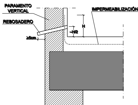
Figura 2.15 Rebosadero
